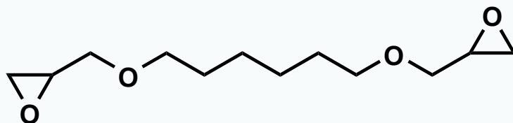
1,6-Hexanediol Diglycidyl Ether
